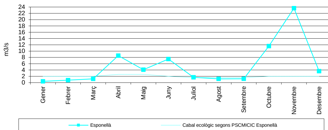
Cabal mensual (2018) - Fluvial Esponellà
