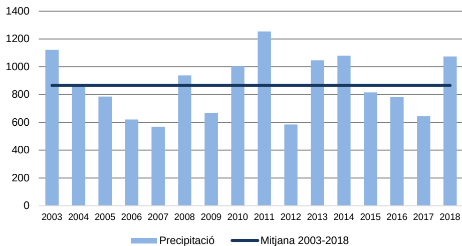
Pluviometria mitjana anual (mm)
